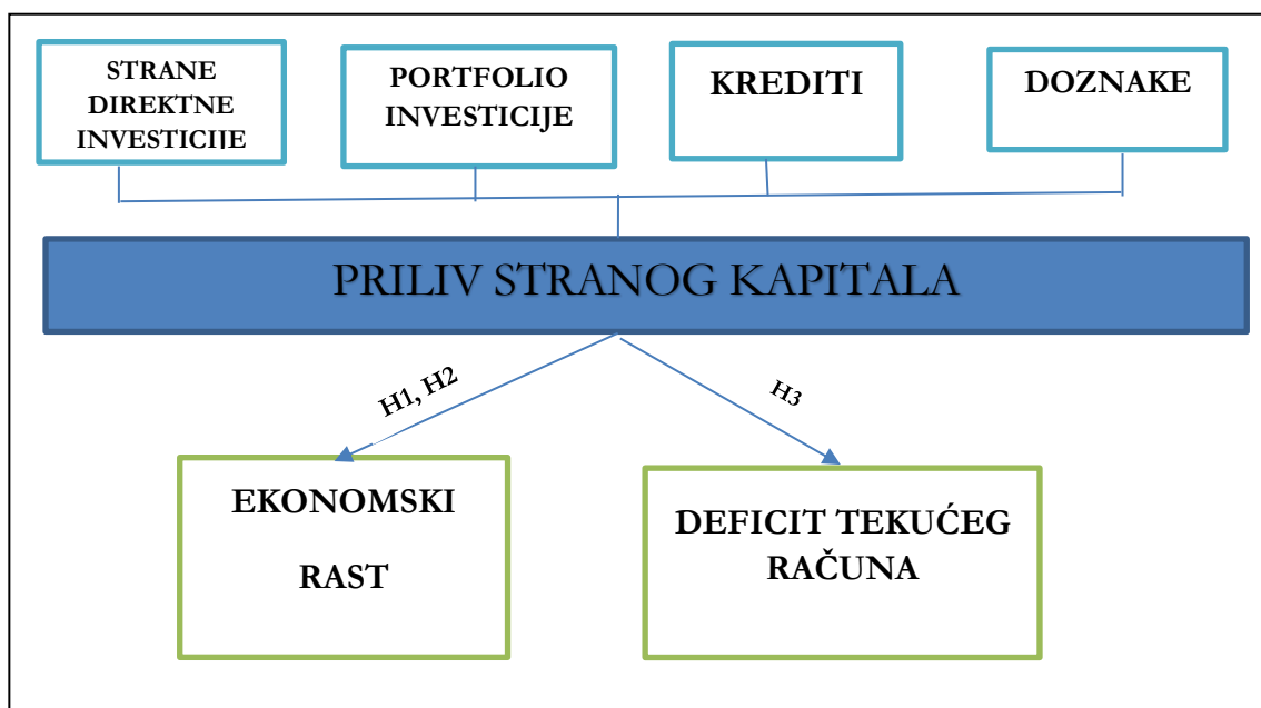
Grafik 1: Istraživački model
